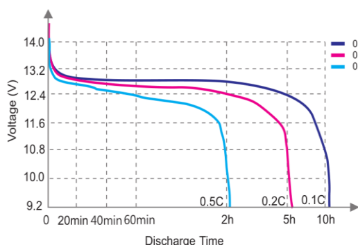
Courbes de décharge de différents courants
